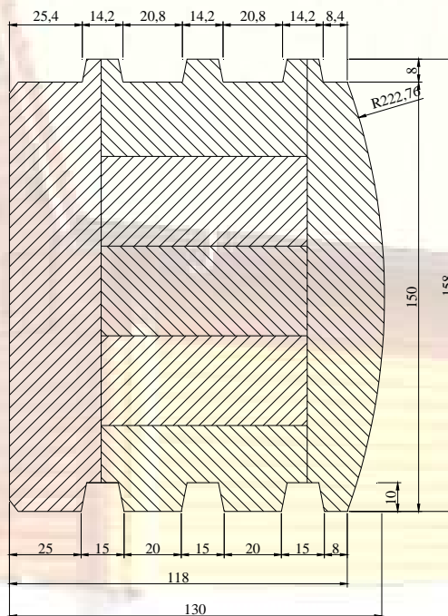
PRESJEK ŠUPLJE GREDE 130/150 mm
